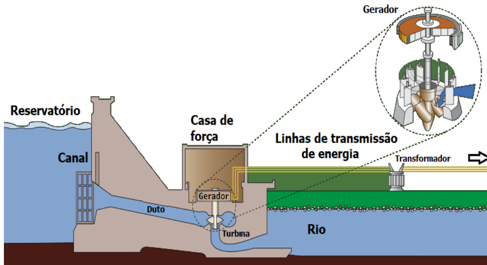
Figura 1 - Usina Hidroelétrica
