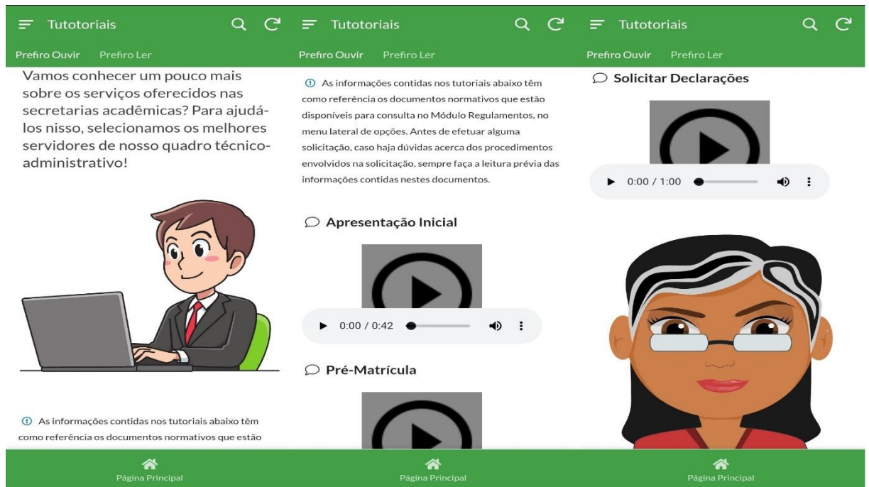
Figura 6 – Módulo Tutoriais
