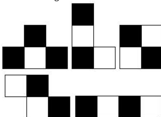
Figura 4: Tetraminó
