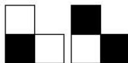
Figura 53: L-triminó
