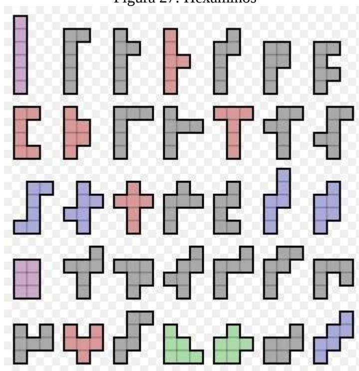
Figura 27: Hexaminós
