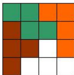
Figura 31: Cobertura 3 tetraminós
