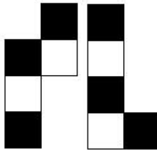
Figura 18: Pentaminós
