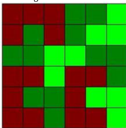
Figura 17: Cobertura
