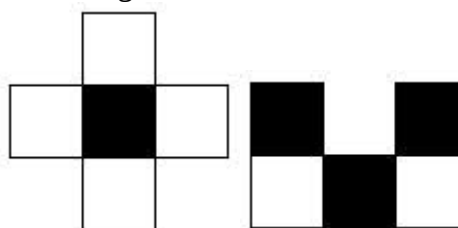
Figura 50: Pentaminós
