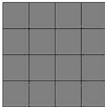
Figura 28: Tabuleiro 4 \times 4
