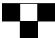
Figura 48: T-tetraminó
