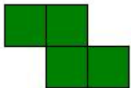
Figura 19: Z-tetraminó
